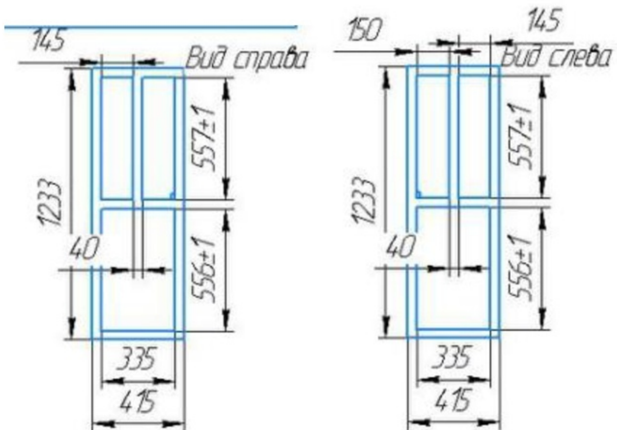
Рисунок 2 Габариты шлагбаума
